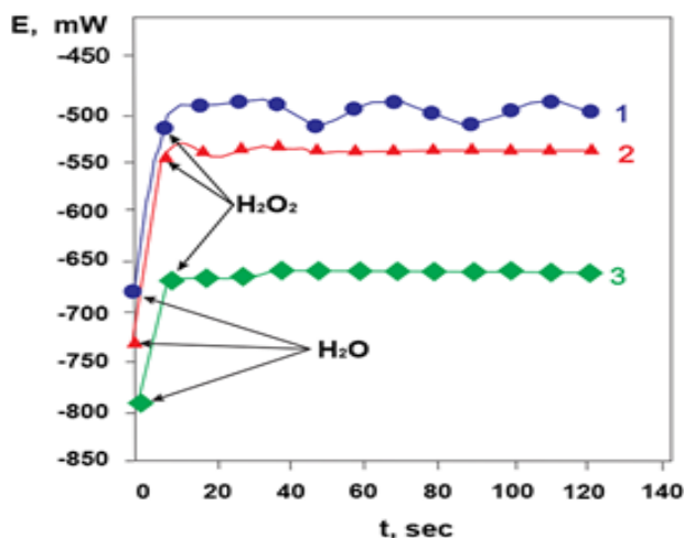
Рисунок 2. Изменение потенциала системы в зависимости от времени: 1- миметический электрод; 2- алюминиевый электрод; 3- алюминиевый электрод с клеем.
