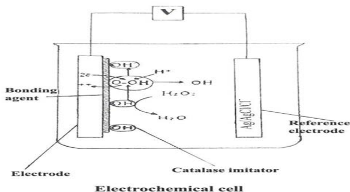
Рисунок 1. Электрохимическая ячейка
