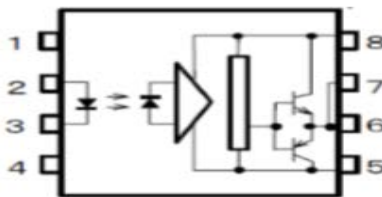
Şəkil 1. TLP250 sürücü qapıları
