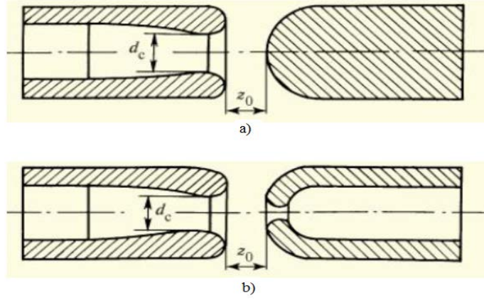
Şəkil 1. SF 6 açarında qövs söndürmə kamerasının görünüşü.
