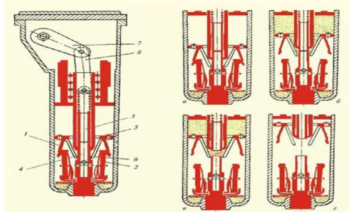
Şəkil 2. Merlin – Gerin firmasının istehsalı olan eleqaz (SF 6 ) açarının kontaktları və açılma mexanizmi.
