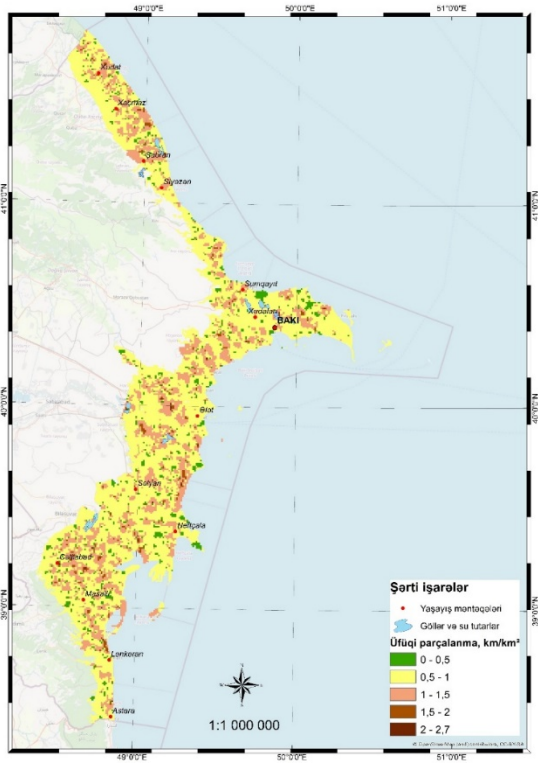
Şəkil 4. Xəzərsahili akkumulyativ düzənliklərin düzənliklərin üfüqi parçalanma xəritəsi
